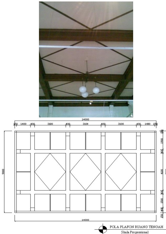
Gambar 14. Pola plafon pada ruang tengah terdapat profil atau lis kayu jati dengan kombinasi bentuk geometris.
