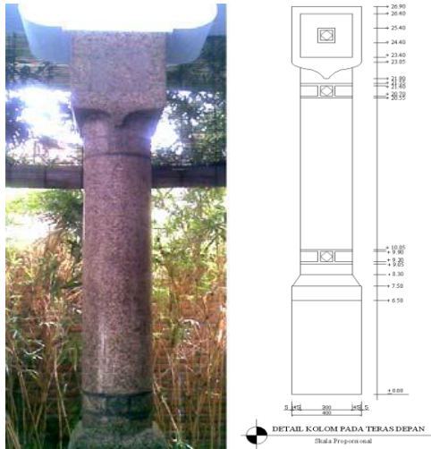
Gambar 5. Detil kolom pada teras depan dengan finishing granit dan juga terdapat detil dekorasi pada bagian badan dan kepala kolom.
