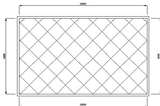
POLA LANTAI TERAS DEPAN Skala Proporsional
