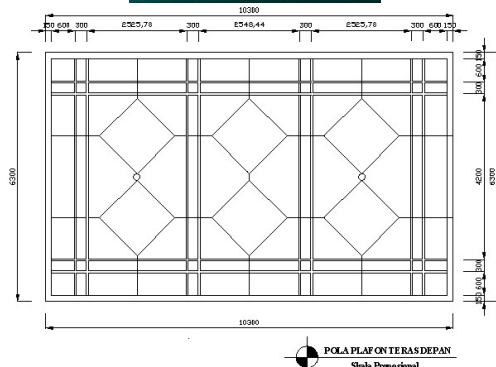
Gambar 7. Pola plafon pada teras depan dengan adanya kombinasi profil kayu dengan bentuk-bentuk geometris
