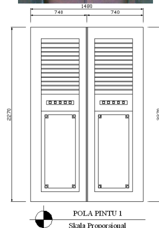
Gambar 16. Pintu 1 pada main entrance yang terbuat dari kayu jati dengan bentuk yang geometris terdapat juga jalusi dan detail dekorasi
