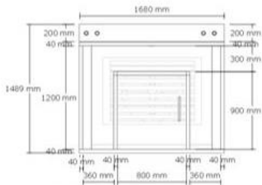
TAMPAK DEPAN SKALA 1 : 20
