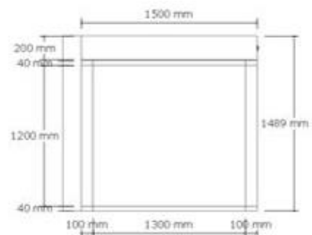
TAMPAK SAMPING SKALA 1 : 20
