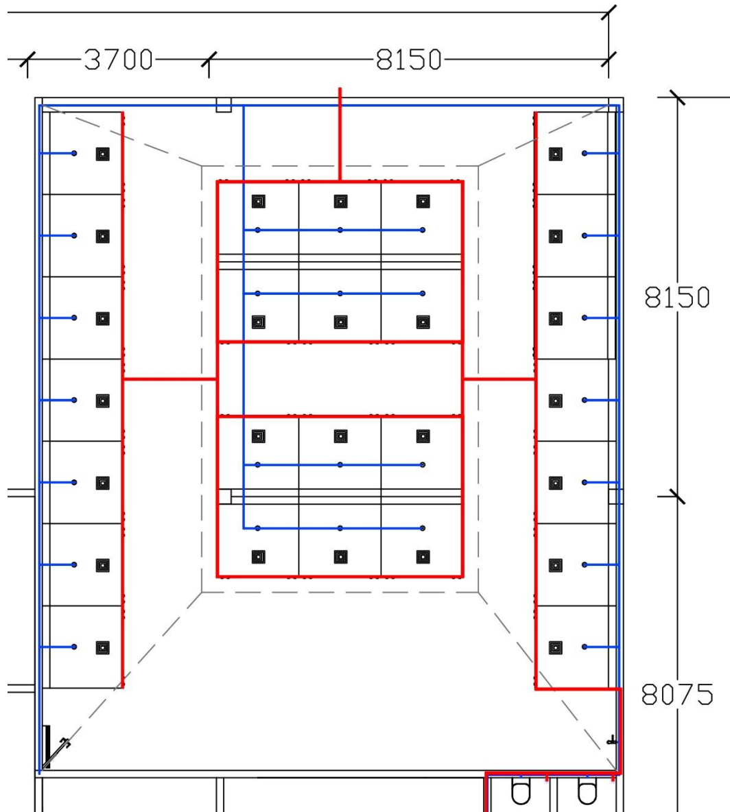
Potongan Tampak Atas Layout Area Penitipan Skala 1:150
